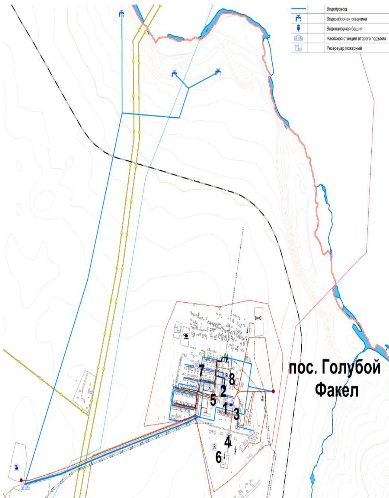
Рисунок №6 Схема водоснабжения пос. Голубой Факел
