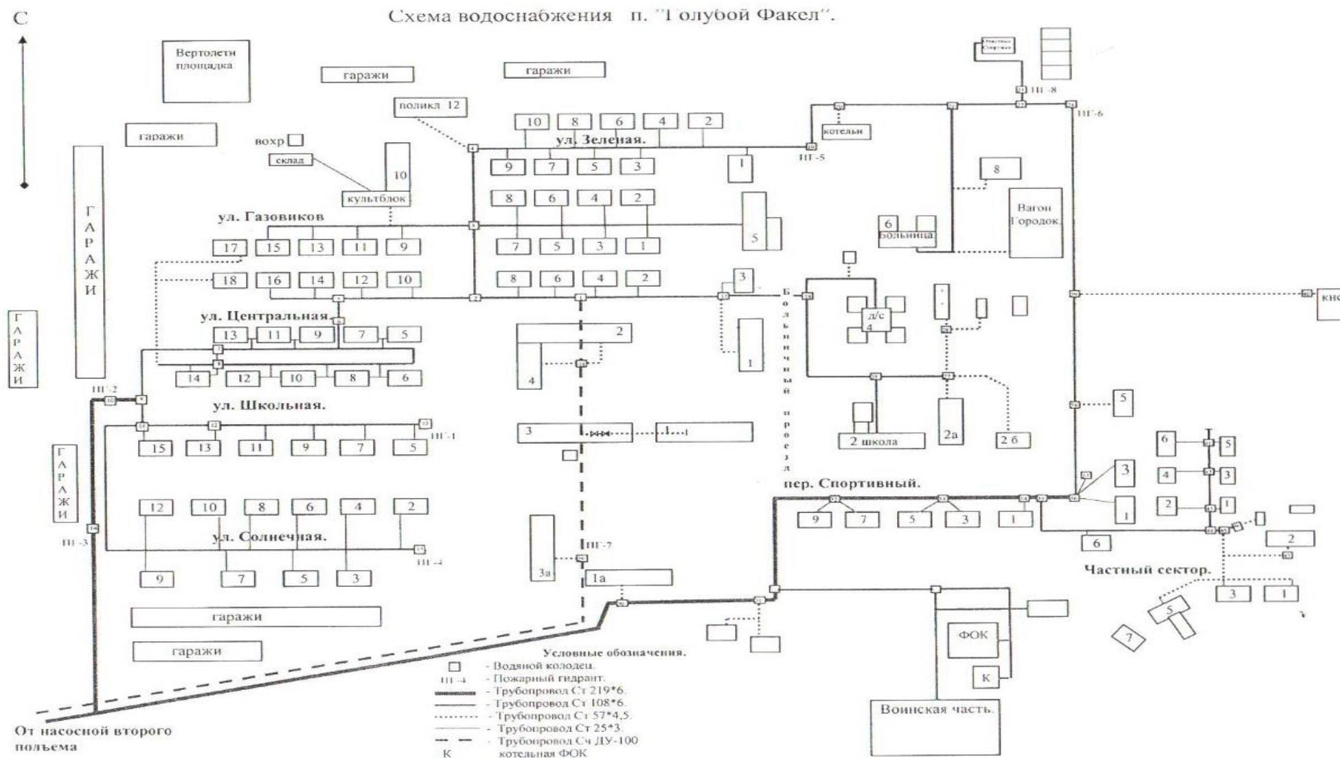
Рисунок №7 Схема водоснабжения пос. Голубой Факел
