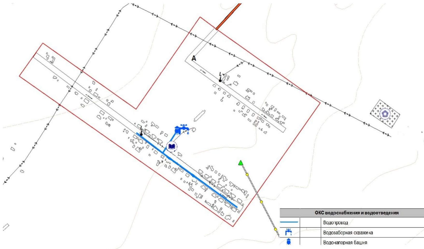
Рисунок №5 Схема водоснабжения с. Камса
